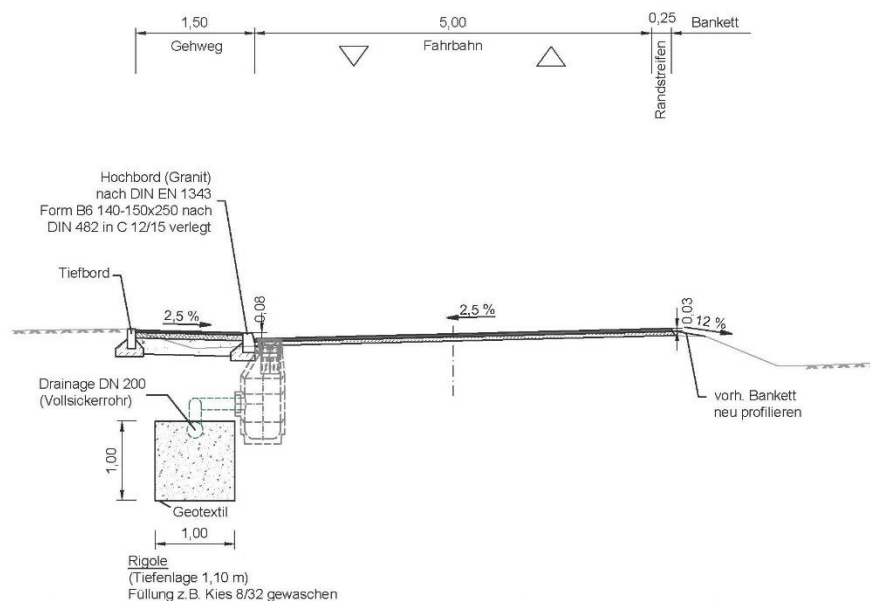
Straßenquerschnitt 1
