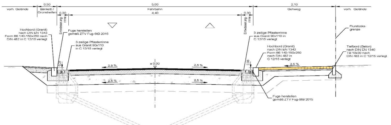
Straßenquerschnitt SQ2
